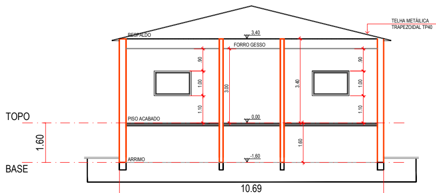
CORTE FF ESC 1:150
