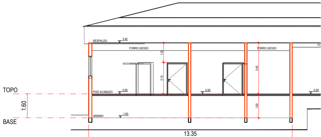
CORTE DD ESC 1:150
