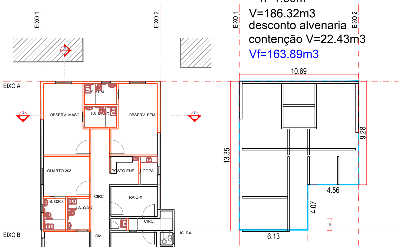
PLANTA BAIXA - CONSTRUÇÃO ESC 1:200
